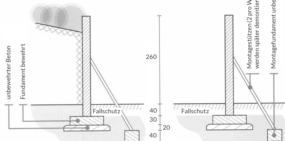
Boulderwand als Böschungswand
