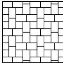
Kreuzverband Bedarf pro m 2 : 24/16/6 - 19,60 Stk. 16/16/6 - 9,80 Stk.
