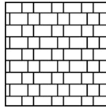
Gotischer Verband Bedarf pro m 2 : 24/16/6 - 15,6 Stk. 16/16/6 - 15,6 Stk.
