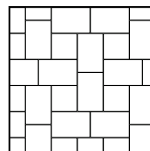
Beispiel 9 Bedarf pro m 2 : 20/20/6 - ca. 6,31 Stk. 30/20/6 - ca. 12,61 Stk.
